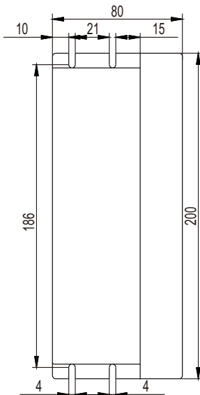
侧面安装图
