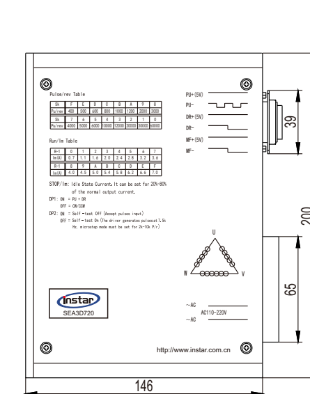
正面安装图
