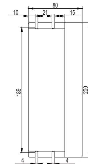
侧面安装图
