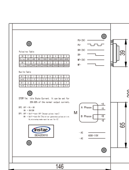
正面安装图
