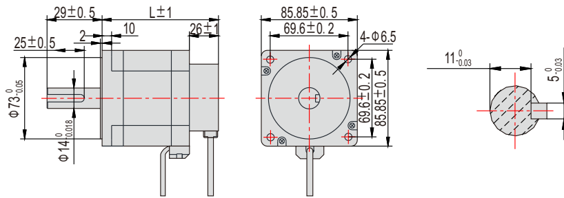
外形图
