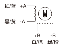
接线图
